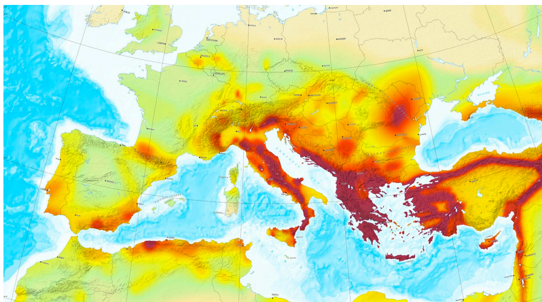
3. ábra Szeizmikus aktivitás a mediterrán régióban (sötét vörös a nagy aktivitás, sárga a mérsékelt, a zöld az alacsony) [3] nyomán
